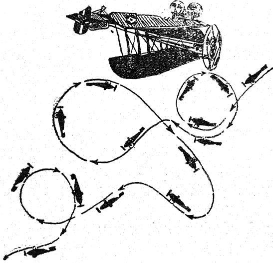
चित्र १७७—वायुयान की फंदेलुमा मंडलाती हुई गति जिसका शिचार्षिकों से अभ्यासकगया जाता है।
